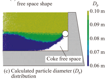
図5 西日本製鉄所(倉敷地区)第4高炉解体調査結果 ((a)黒鉛化度分布, (b)充填層構造とコークスフリースペース, (c)粒度 ( D_p ) 分布計算結果) Fig.5 Dissection analysis Results of No. 4 blast furnace, West Japan Works (Kurashiki)
