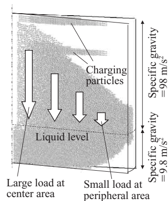
図2 堆積粒子と大重力による荷重分布再現
