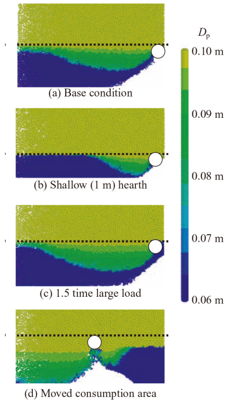
図9 炉床コークス粒度分布計算結果 ((a) ベース条件 (b) 炉床浅い (1 m), (c) 荷重 1.5 倍, (d) 消費位置変更) Fig.9 Calculated result of coke diameter distribution in hearth
