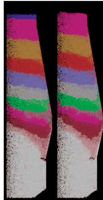
(a) 1.2 m (b) 1.5 m 図7 レースウェイ位置の炉芯サイズへの影響の計算結果 Fig.7 Calculated effects of raceway position on dead man size by DEM
